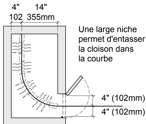
Fermeture sur porte de niche
