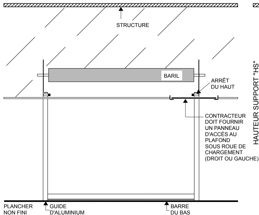
ÉLEVATION CÔTÉ BARIL ( INTÉRIEUR )
