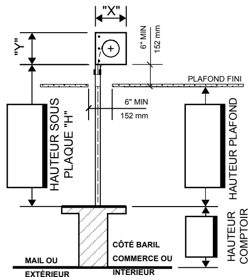
COUPE ( COMPTOIR )
