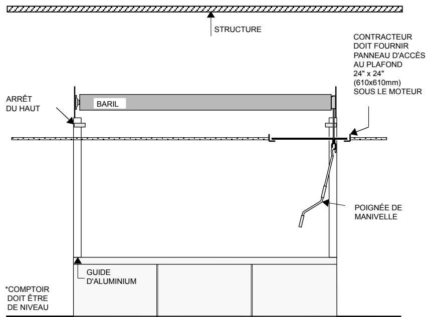
( INTÉRIEUR ) ÉLEVATION CÔTÉ BARIL
