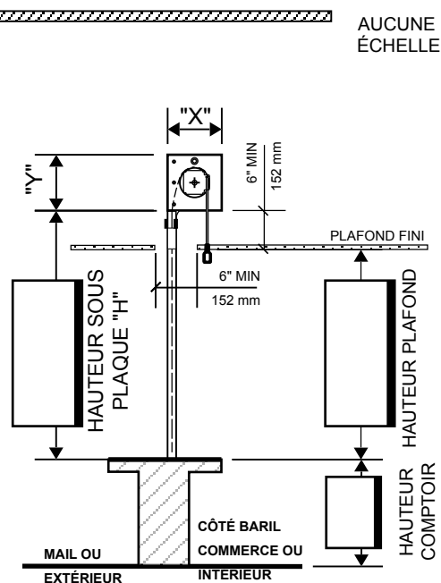
COUPE ( COMPTOIR )
