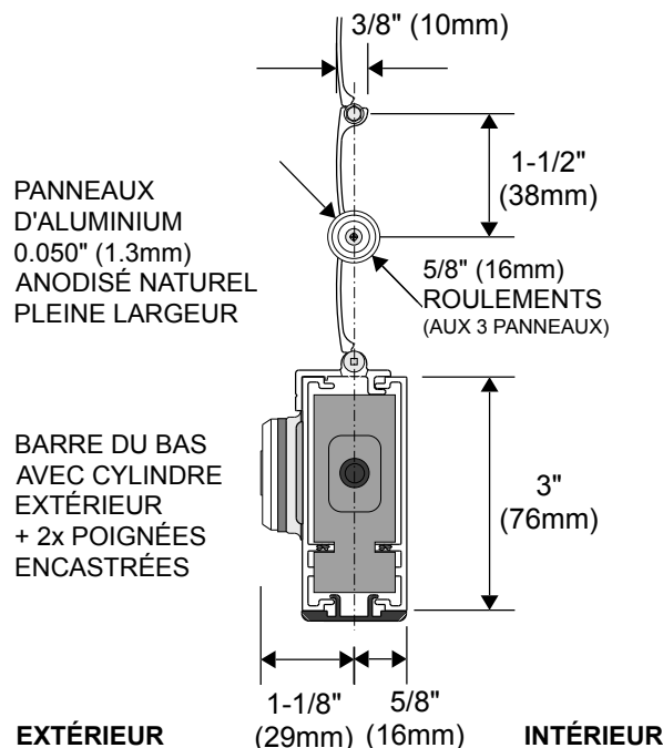
COUPE ( RIDEAU ET BARRE DU BAS )
