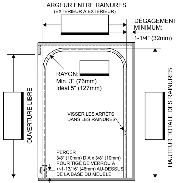
COUPE ( MEUBLE )
