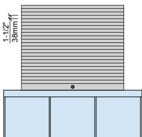
COUNTER SHUTTER (Opaque)
